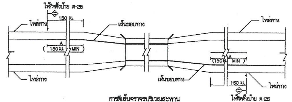
การติดตั้งจากรอบบริเวณสะพาน
