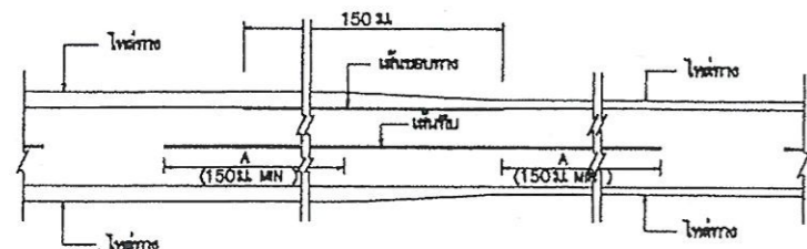
การติดตั้งจากรอบบริเวณโค้งราบ กรณีความกว้างของไหล่ทางลดลง
