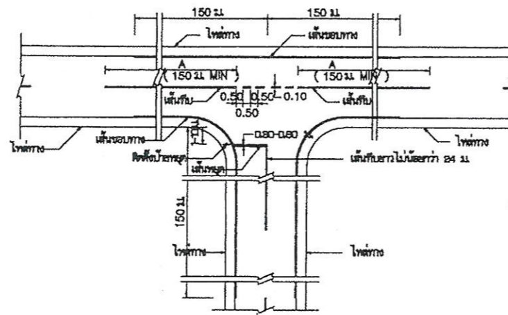
การติดตั้งจากรอบบริเวณแยก
