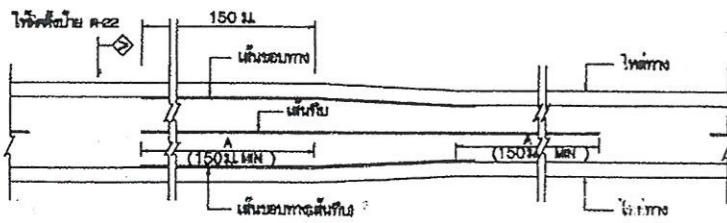
การติดตั้งจากรอบบริเวณโค้งราบ กรณีความกว้างของช่องจราจรลดลง
